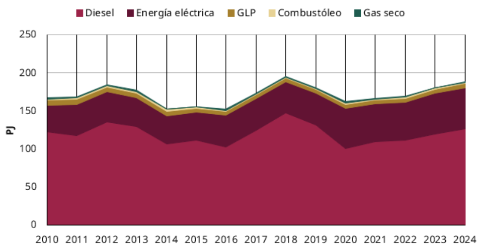
Figura 24. Figura 5.4 Evolución del consumo energético del sector agropecuario por energético, 2010-2024
