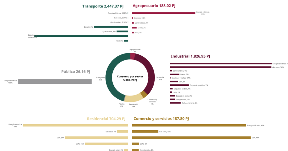
Figura 42. Figura 6.5 Estructura del consumo final por sector y energético, 2024
